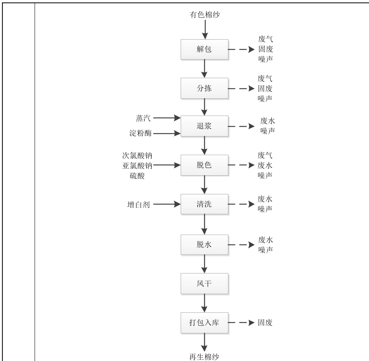
图2-3 再生棉纱工艺流程和产污环节分析图
