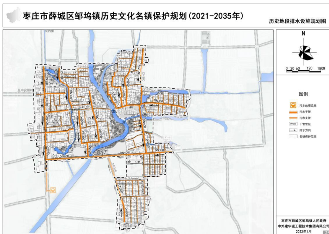
图 8-16 历史地段排水设施规划图
