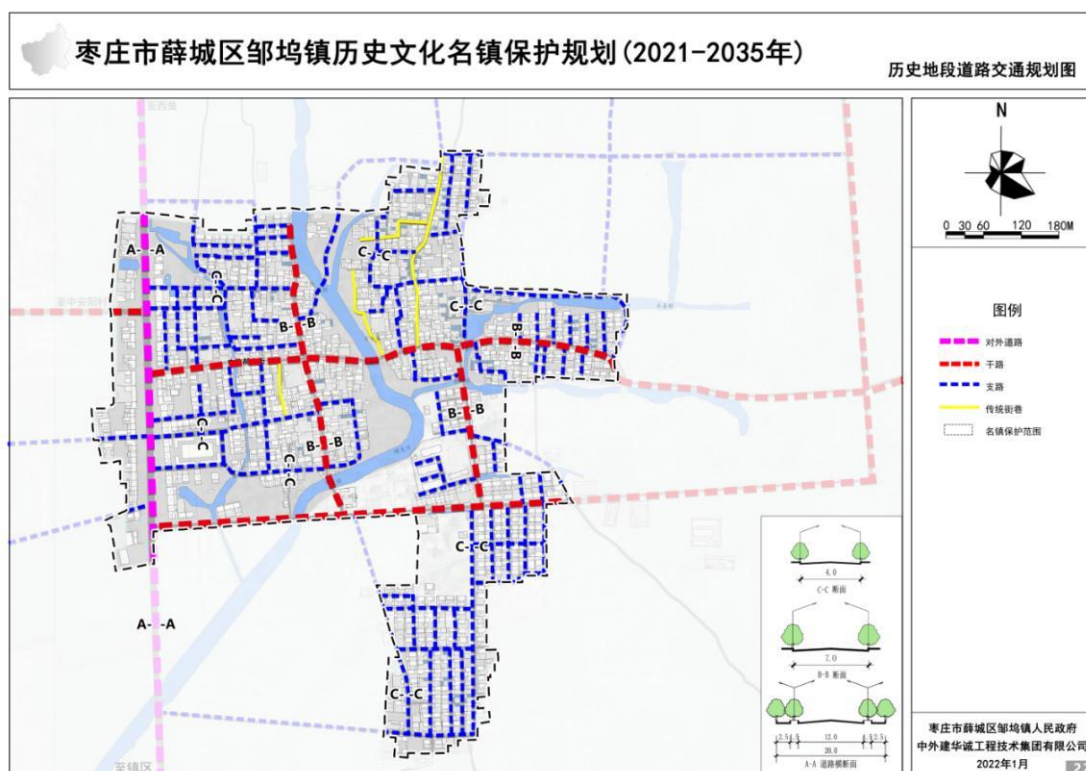
图 8-14 历史地段道路交通规划图
